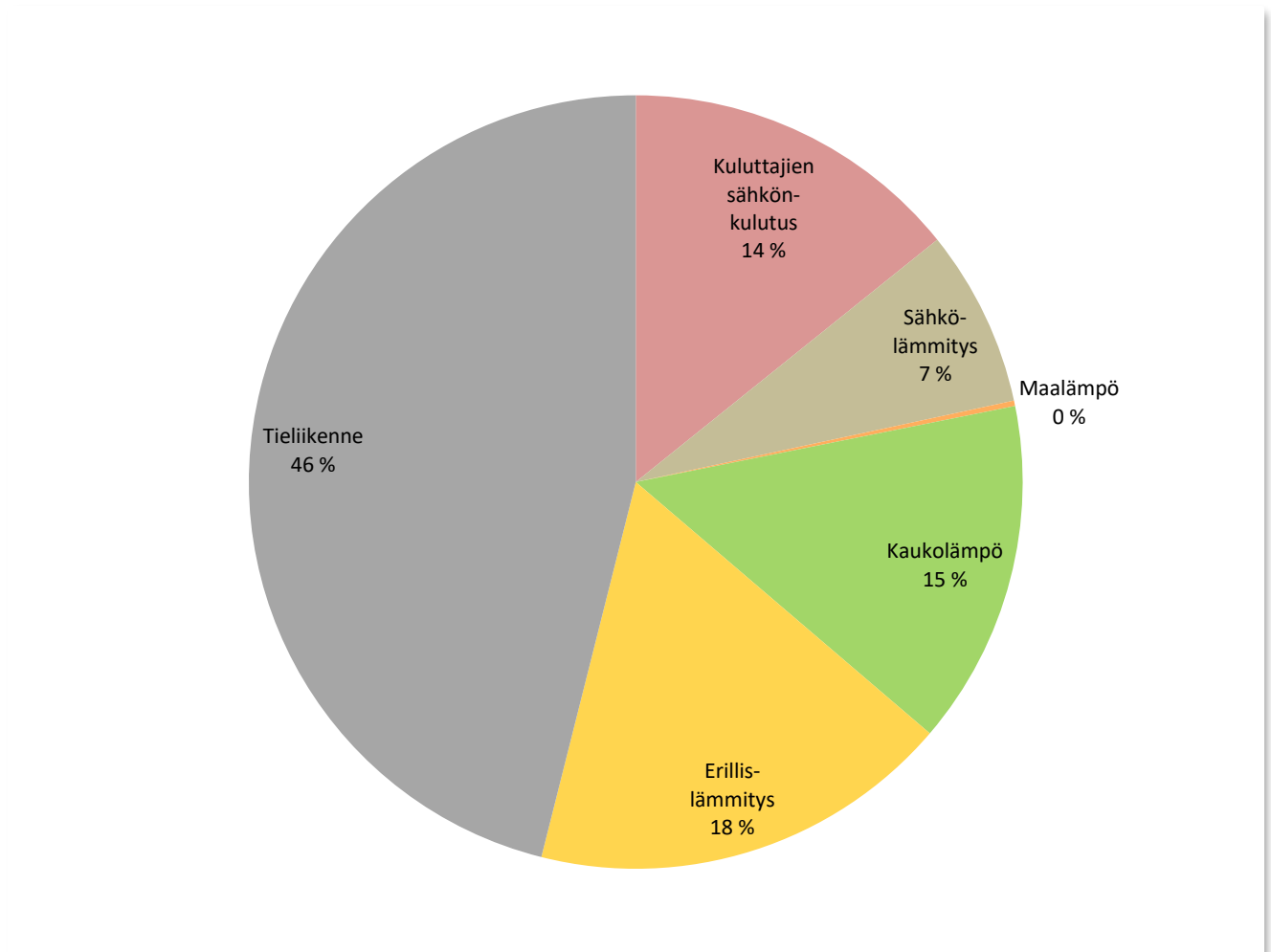
Kuva 13. Energian loppukulutuksen jakautuminen eri sektoreille Paimiossa vuonna 2016 ilman teollisuutta. Energian loppukulutus ei sisällä lämpöpumppujen tuottamaa uusiutuvaa energiaa, mutta sisältää niiden käyttämän sähkön.
