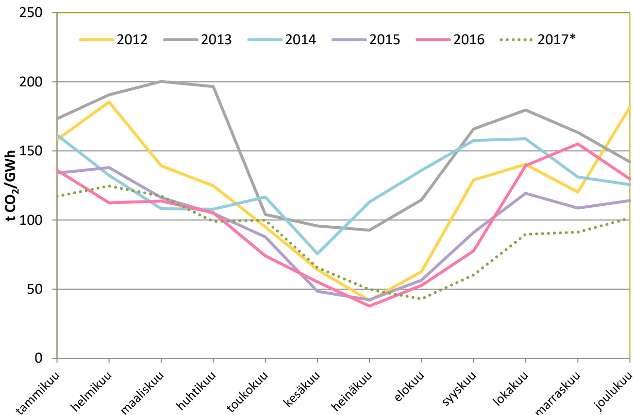
Kuva 1. Sähkönkulutuksen päästökerroin kuukausitasolla vuosina 2012–2017, laskettuna hyödynjakomenetelmällä Energiategollisuus ry:n aineistosta. Vuoden 2017 tieto on ennakkotieto.
