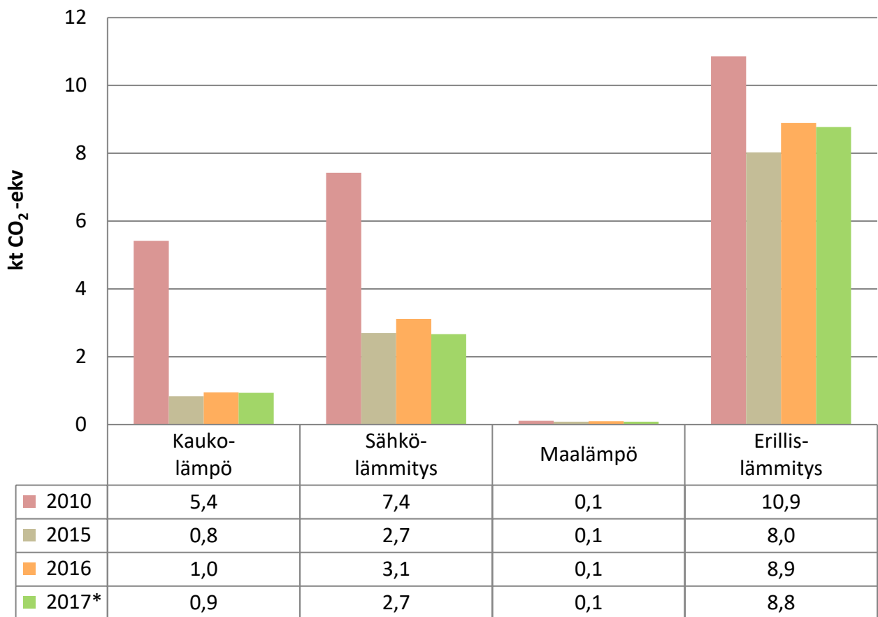
Kuva 6. Rakennusten lämmityksen päästöjen kehitys Paimiossa vuonna 2010 ja vuosina 2015–2017. Vuoden 2017 tieto on ennakkotieto.
